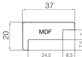
DETTAGLIO TECNICO
